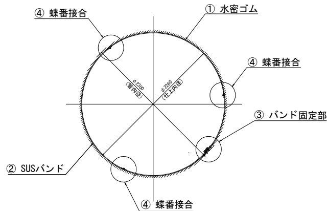
組立図
