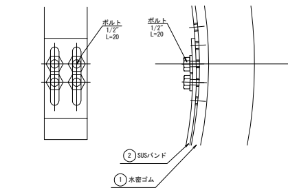
③ SUSバンド固定部詳細図
