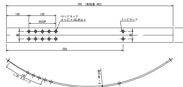
調整バンド詳細図
