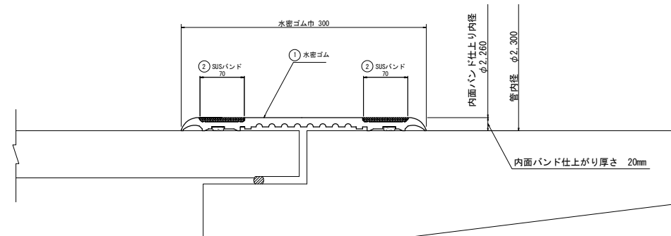
断面図
