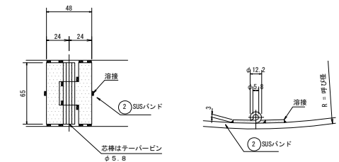
④ 蝶番接合詳細図
